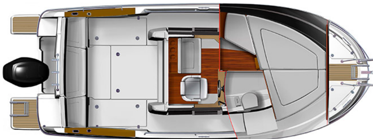
План нижней палубы
